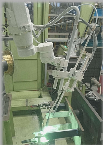
半自動ろう付け設備
