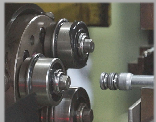
ロール（溝）成形
