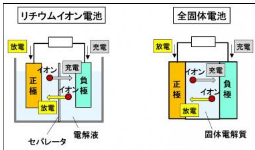
【図表 1】リチウムイオン電池と全固体電池の構造（出所：自動車用語辞典 HP より）
